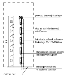
DETAL "A" BALUSTRADY PRZY SALI GIMNASTYCZNEJ 1:20
