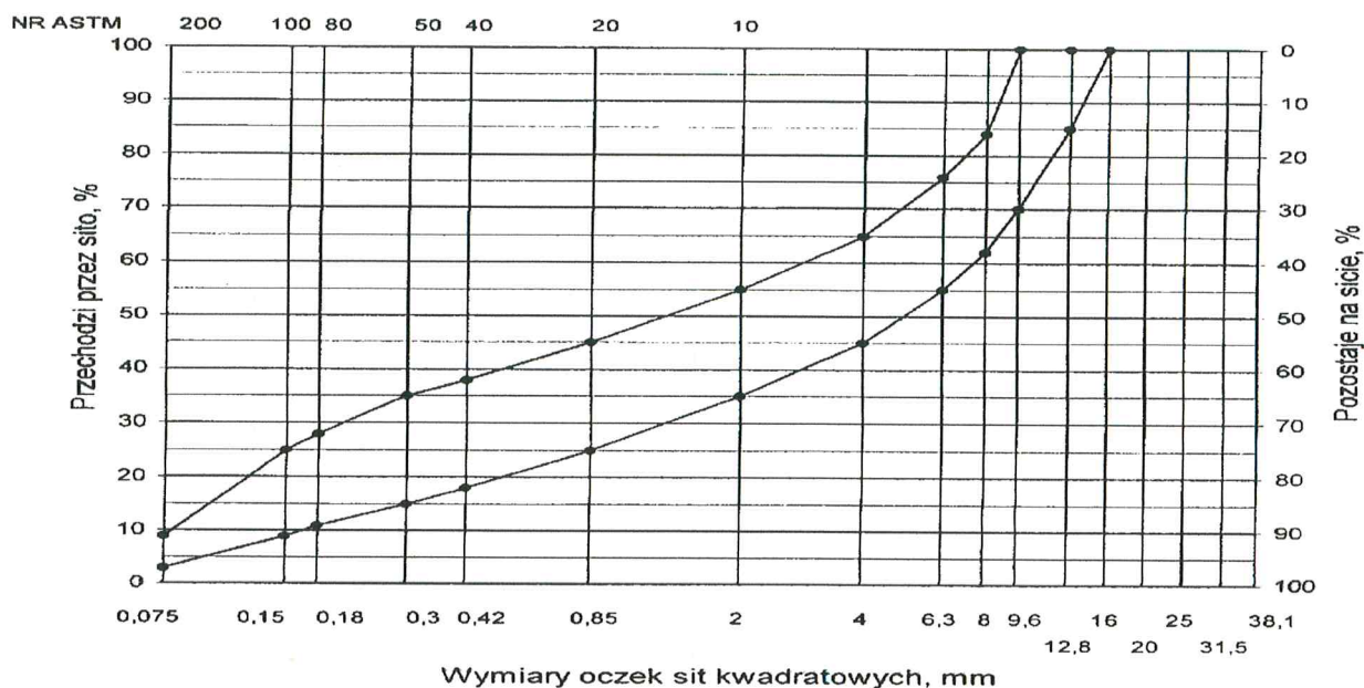
Rys. 10. Krzywe graniczne uziarnienia mieszanki mineralnej BA od 0 do 12,8 mm do warstwy wiążącej, wyrównawczej i wzmacniającej nawierzchni drogi o obciążeniu ruchem KR1 lub KR2
