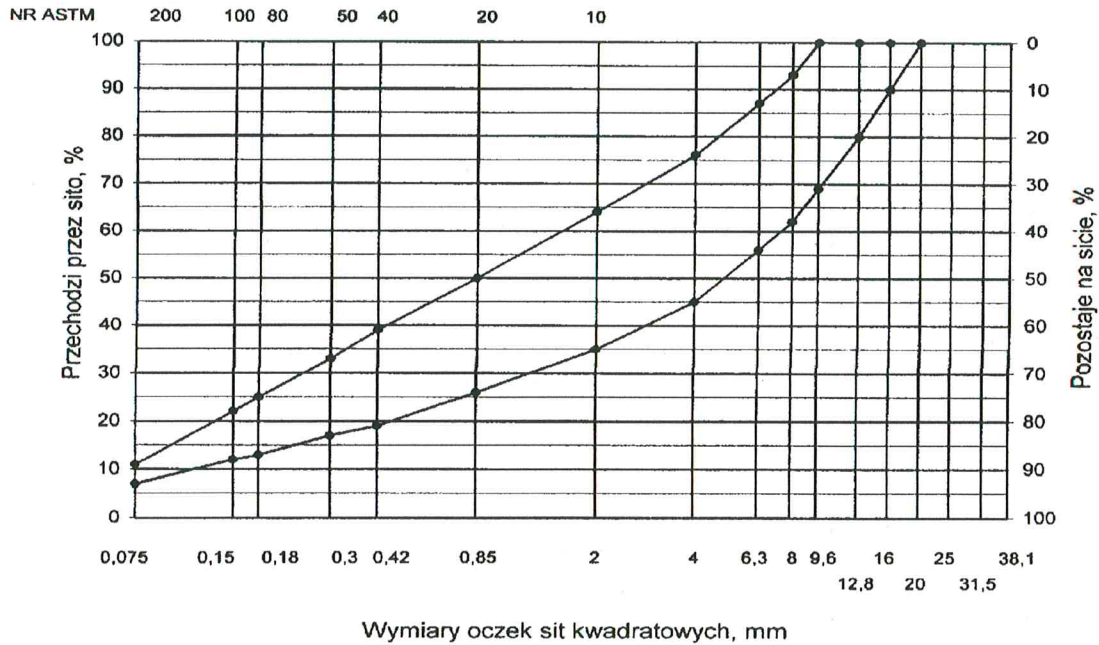
Rys. 2. Krzywe graniczne uziarnienia mieszanki mineralnej BA, od 0 do 12,8 mm do warstwy ścieralnej nawierzchni drogi o obciążeniu ruchem KR1 lub KR2
