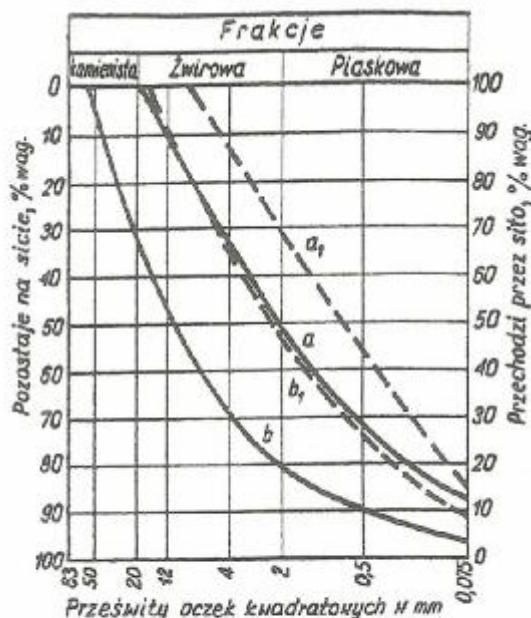
Rysunek 1. Obszar uziarnienia optymalnych mieszank żwirowych
